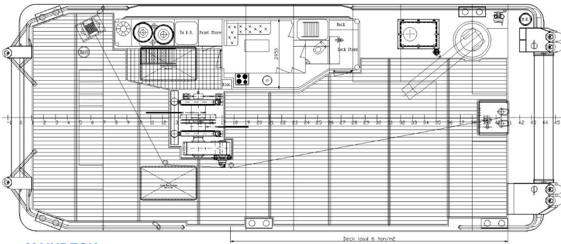
MAINDECK
